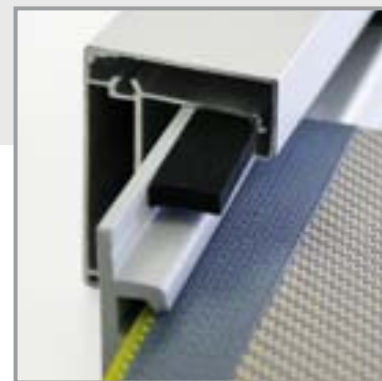
DETAIL SEITENFÜHRUNG
